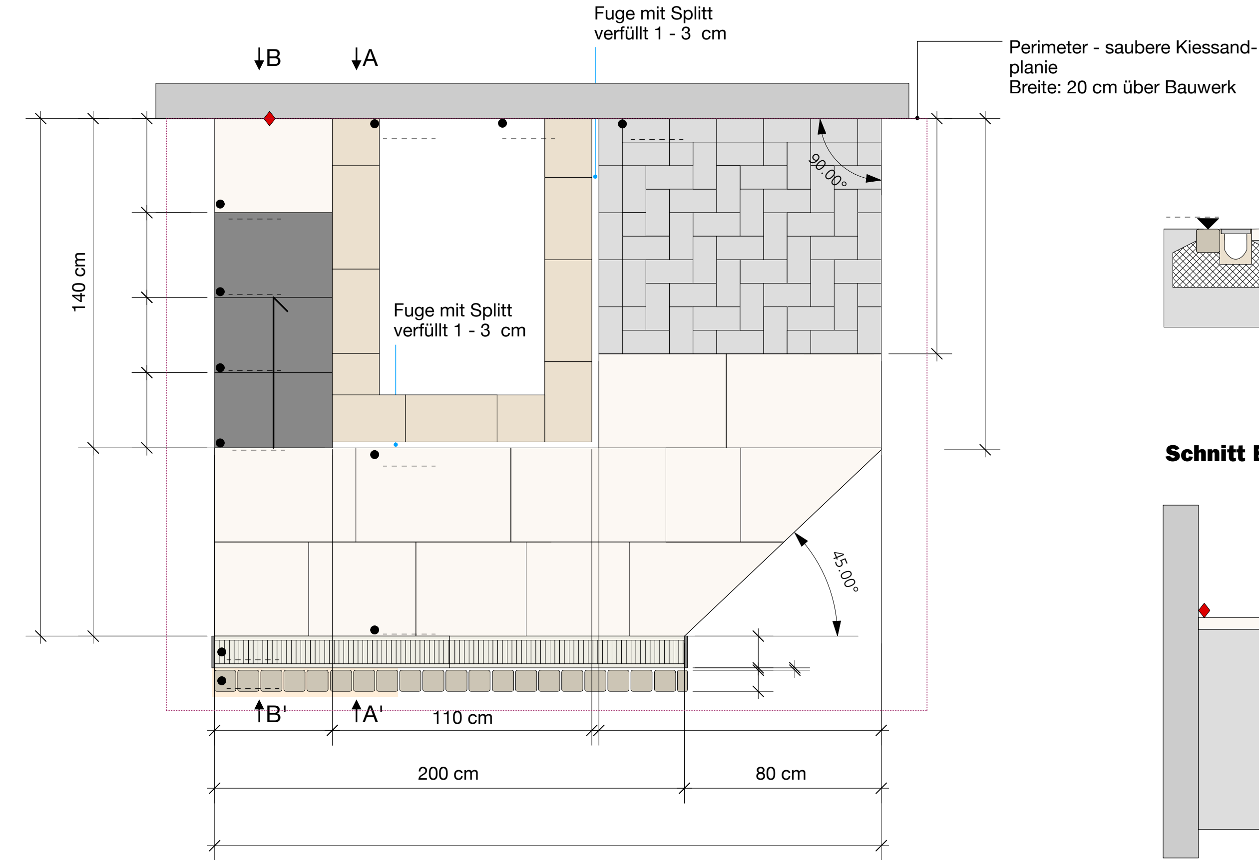
Grundriss M 1:20
