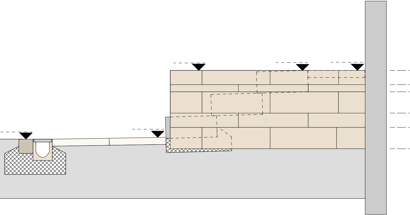
Schnitt A - A' M 1:20
