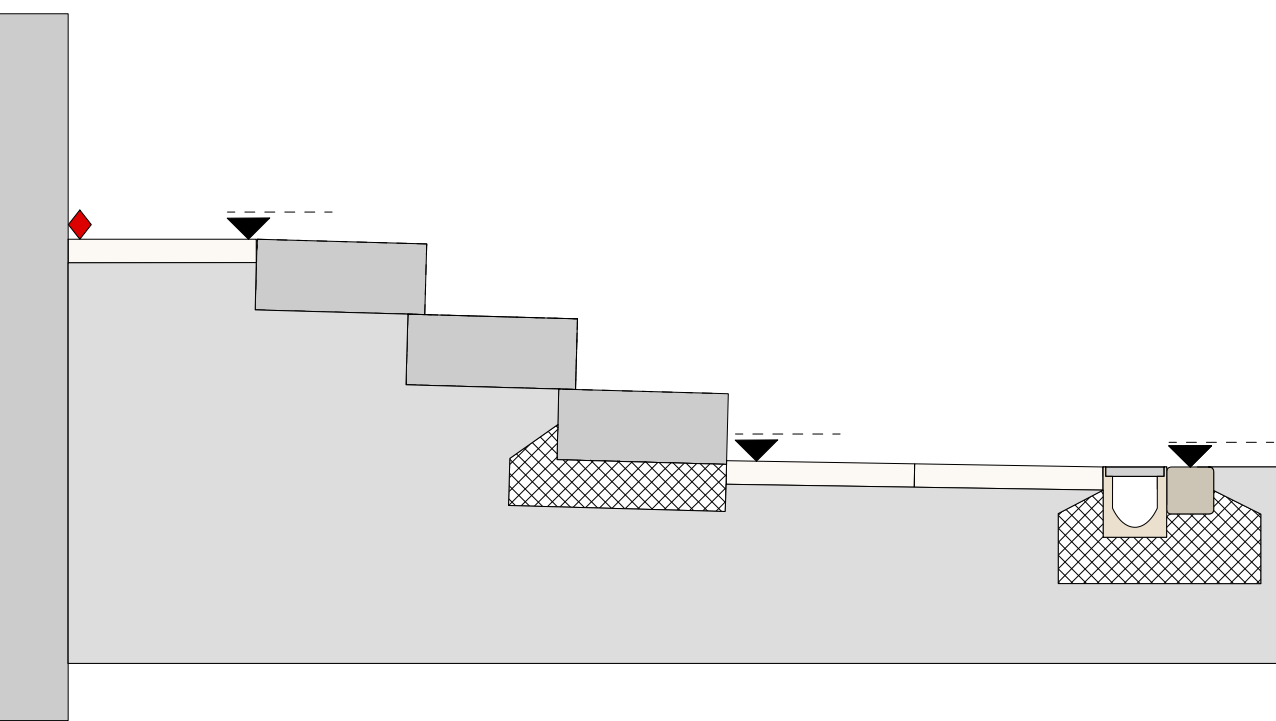
Schnitt B - B' M 1:20
