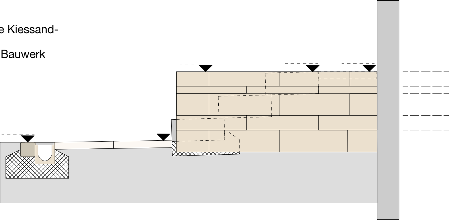
Schnitt A - A' M 1:20
