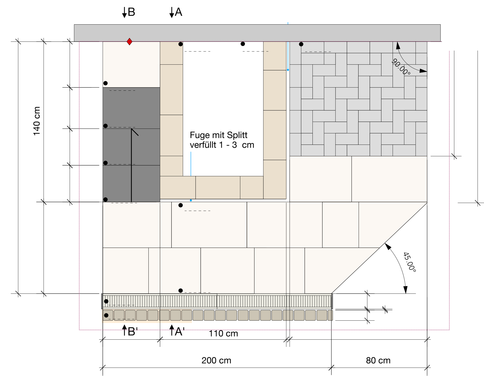
Grundriss M 1:20
