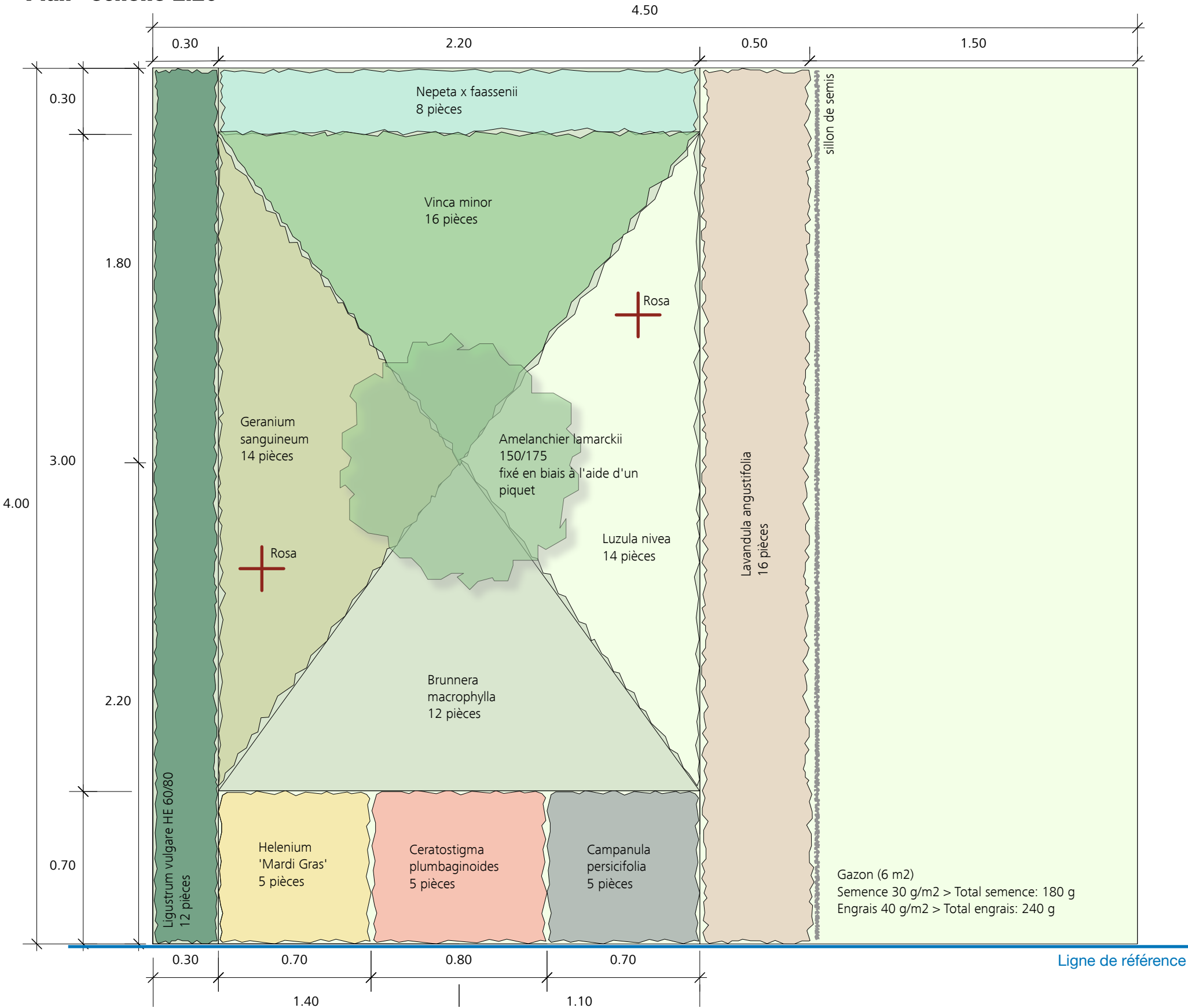
Plan - échelle 1:20
