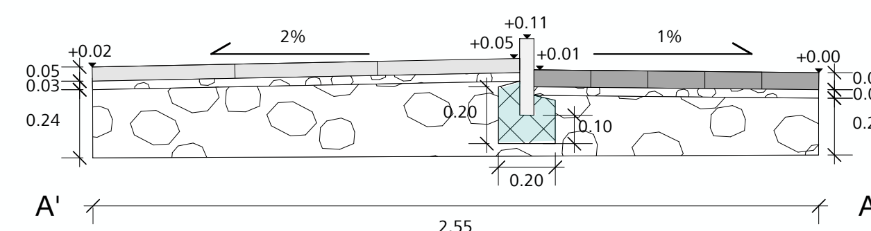
Coupe A - A' - échelle 1:20
